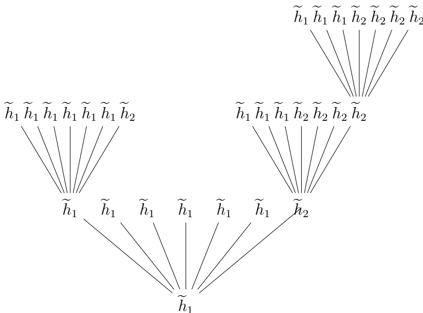
РИС. 1. Совокупность векторов h_x , построенных по правилам (l_1) на дереве Кэли порядка k = 7 .
