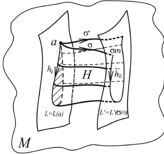
Рис. 2.2: Кривая \sigma' \in \Omega_a — результат действия элемента [h_0] \in \pi_1(L, a) на кривую \sigma \in \Omega_a
